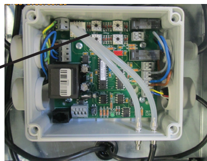
Рис. 4: Задание уставки дифференциального давления с помощью переключателей
