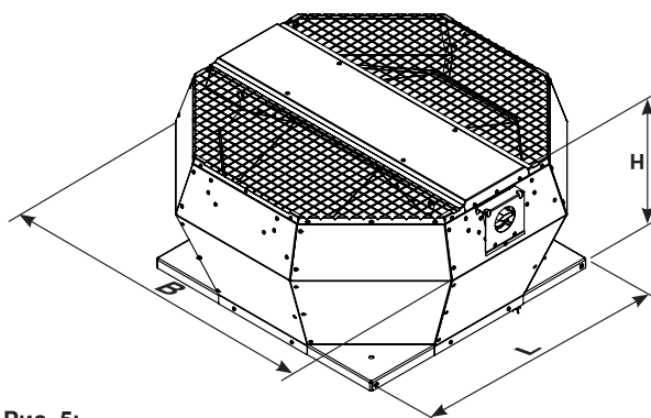
Рис. 5: Размеры агрегата
