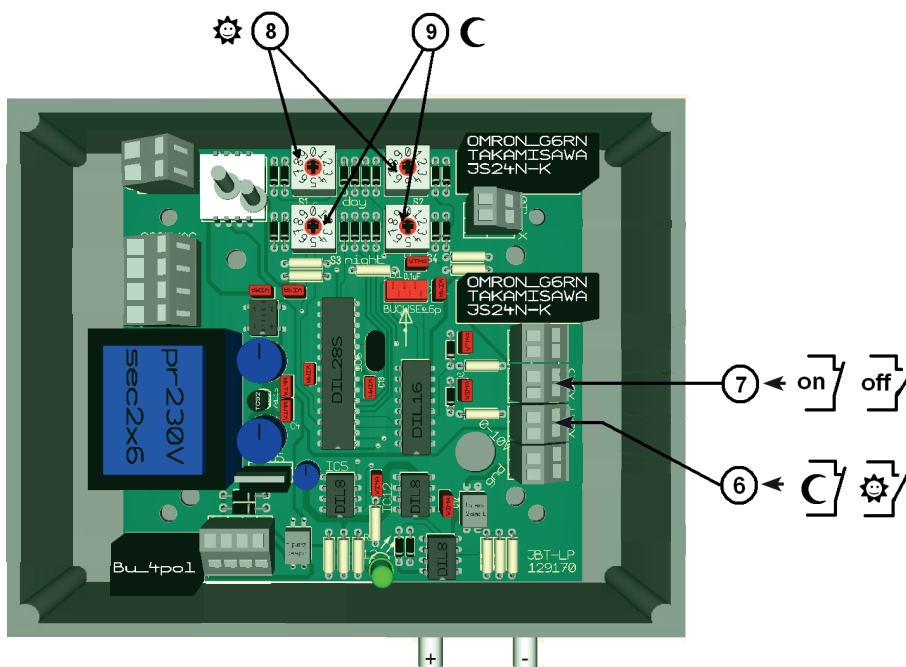
Рис. 3: Зажим для подключения устройства управления
