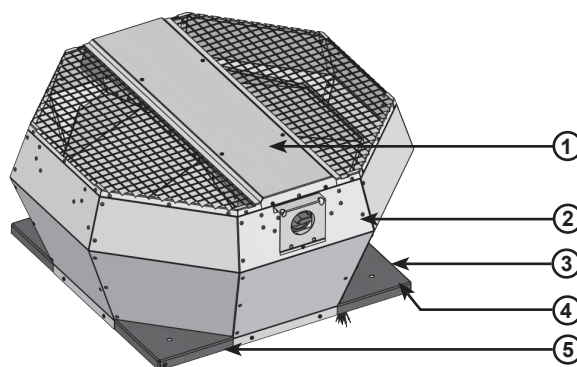
Рис. 1: Крышный вентилятор
